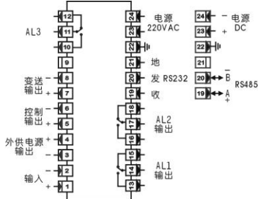
接线端子图
