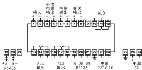
接线端子图
